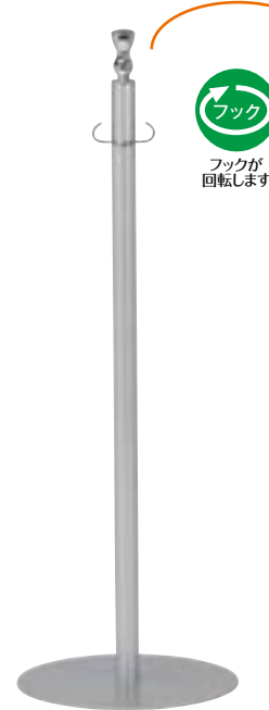
PS-407 ¥21,000 S:300φ×H875mm(ポール32φmm) C:クローム/シルバー塗装 重量:3.3kg Lot:1 ★ポール:真鍮+スチール ベース:スチール
