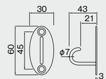
フック PR-6 1本¥1,700 S:60×30×43mm ★ロープは別売
