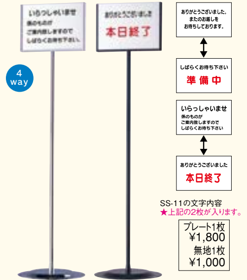
SS-11 インフォメーションスタンドA-4(ヨコ) S:300φ×H1113mm、Lot:1 C:ブラック ¥27,000 C:クローム ¥32,000 ★プレート2枚差し
