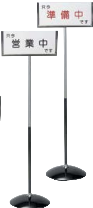
営業中/準備中 SS-221 ¥29,000 S:279φ×H1177mm C:上部クローム・ 下部ブラック、Lot:1 ★表 営業中/裏 準備中 ボード4mm
